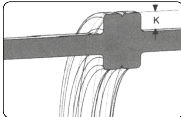
Şekil 6: Dudak detayı
